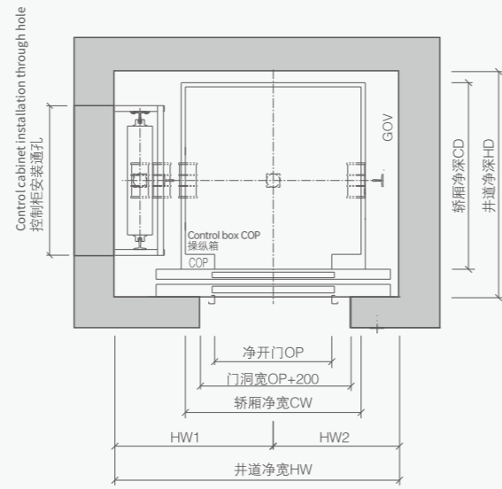
井道平面图 Hoistway plan
