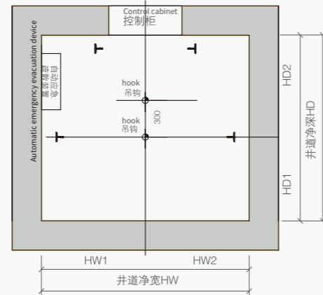
吊钩图 Hook detail
