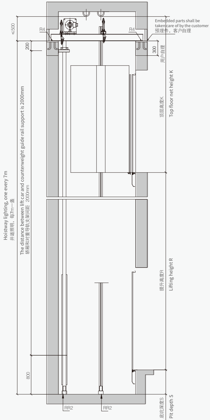
井道立面图 Elevation
