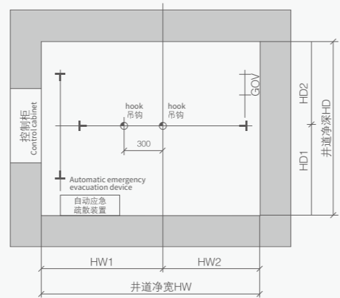
吊钩图 Hook detail
