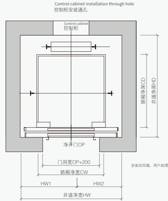
井道平面图 Hoistway plan
