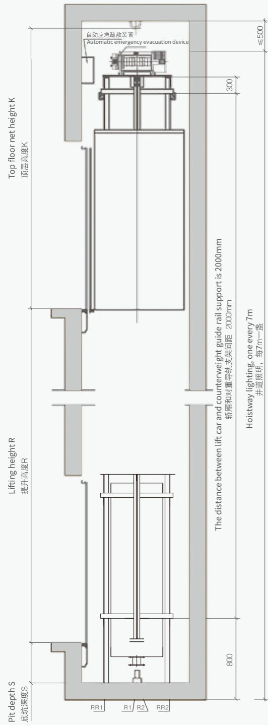
井道剖面图 Elevation
